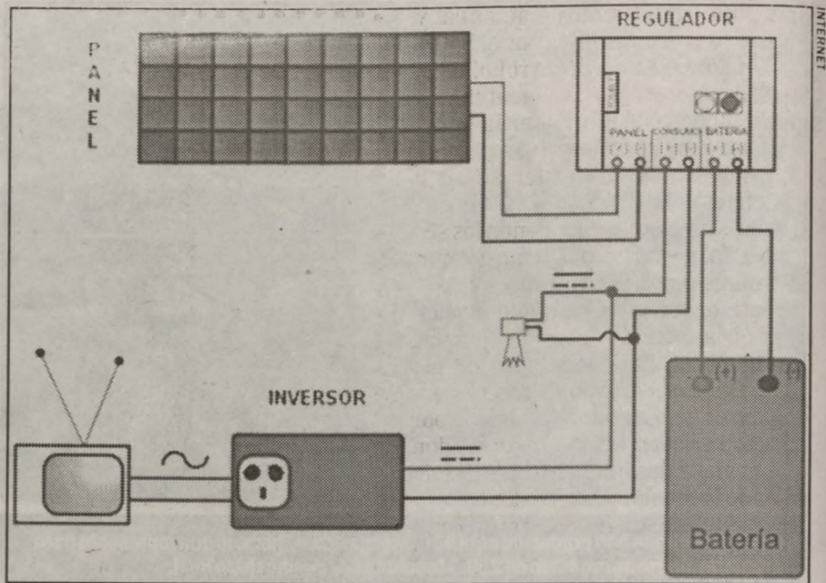
Esquema que ilustra la generación fotovoltaica, su distribución y consumo.
